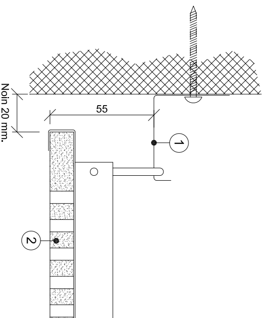
LEIKKAUS A-A
